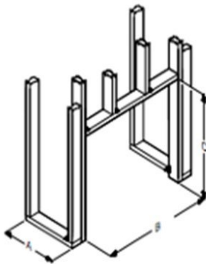
Rohbau Rahmenmaße
